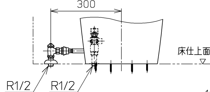
正面図 床給水仕様の場合
